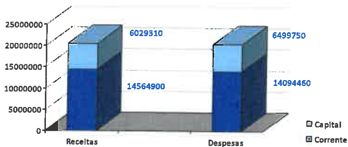
Figura 1 – Saldo Corrente
